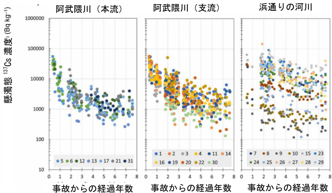
図3：2011～2019年における県内河川の懸濁態 ^{137}\text{Cs} の減少（提供：福島県）
