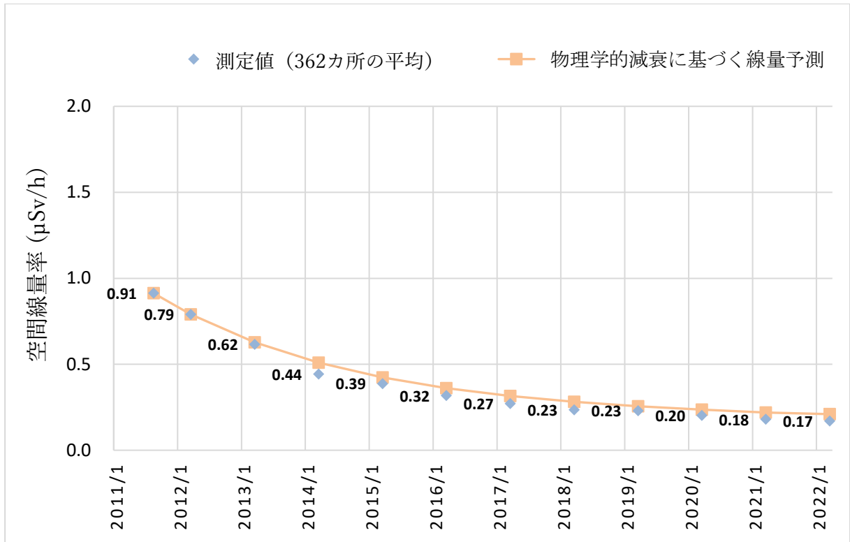
図1：2022年までの県内の森林における362カ所のモニタリング地点の空間線量率及び放射性セシウムの物理学的減衰に基づく空間線量率の予測（提供：福島県）
